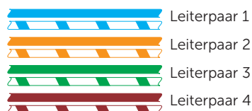
Abb. 29 Farbcode und Zählweise eines Netzkabels (EIA/TIA-568B)
