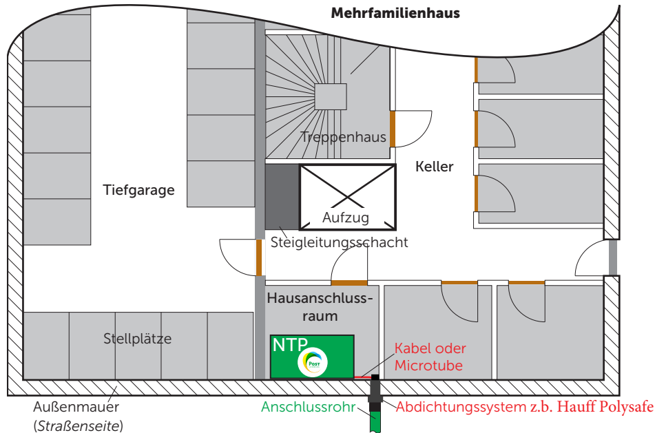
Abb. 1 Hausanschlussraum mit direktem Kontakt zum Anschlussrohr
