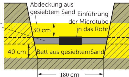
Abb. 9 Einführung der Microtube in das Rohr in der Anschlussgrube mit Schutz des Rohres und der Microtube mit einer Abdeckung aus gesiebttem Sand
