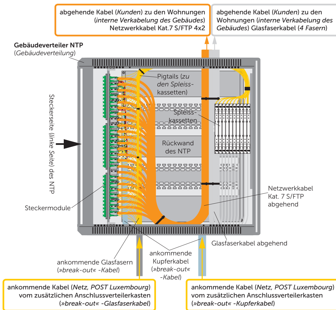
Abb. 24 Gebäudeverteiler NTP – (Verteilung des Gebäudes, Frontansicht) ohne Tür
