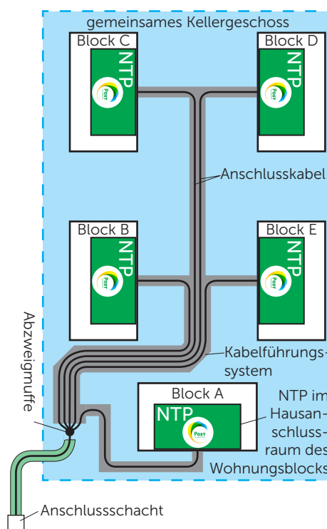
Abb. 4 Gemeinsamer Anschluss von allen Wohnungsblöcken
