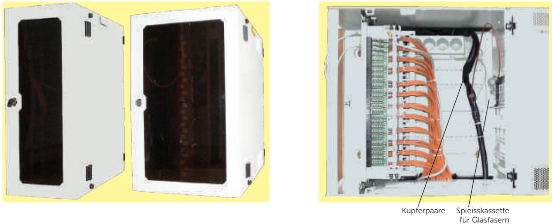
Abb. 21 Verschiedene Typen von NTP von POST Luxembourg (4 HE und 6 HE) – rechts NTP geöffnet
