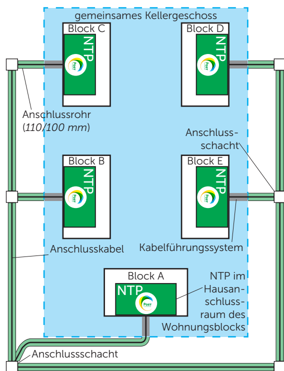
Abb. 3 Individueller Anschluss eines jeden Wohnungsblocks
