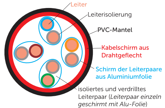
Abbildung 27 Netzkabel Kat.7 S/FTP 4x2 (Paare geschirmt) für die Vertikalverkabelung
