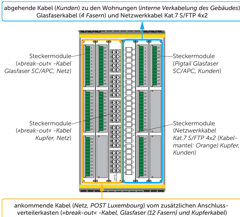
Abb. 23 Gebäudeverteiler NTP Steckerseite (linke Seite, Seite für die Patch-Verbindungen), ohne Tür
