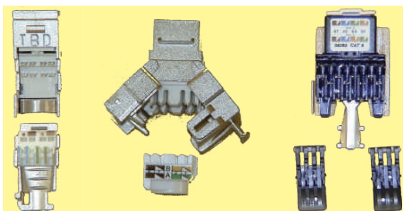
Abbildung 33 Verschiedene Typen von Anschlussmodulen RJ45 Kat.7 und Kat.6
