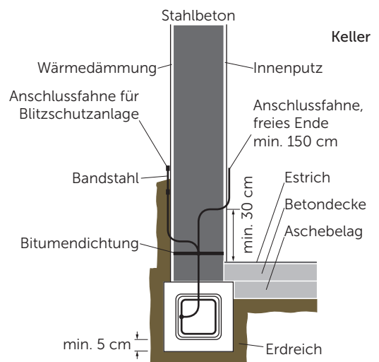
Abb. 19 Erdungsanlage Typ B, Fundamenteerder
