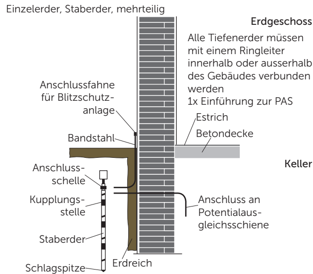
Abb. 17 Erdungsanlage Typ A, Einzelerder
