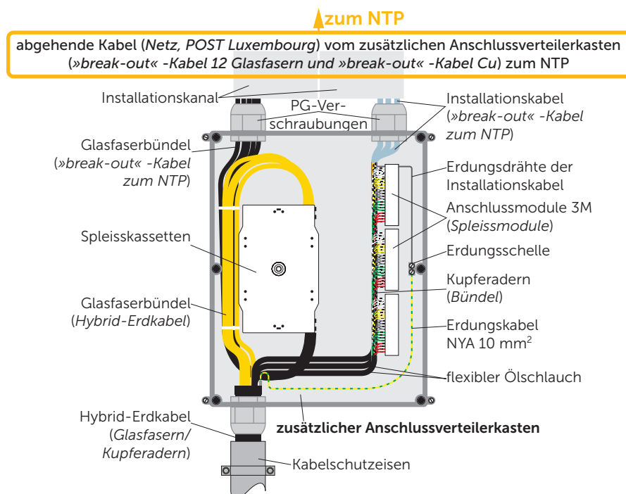
Abb. 22 Zusätzlicher Anschlussverteilerkasten (unter dem NTP)
