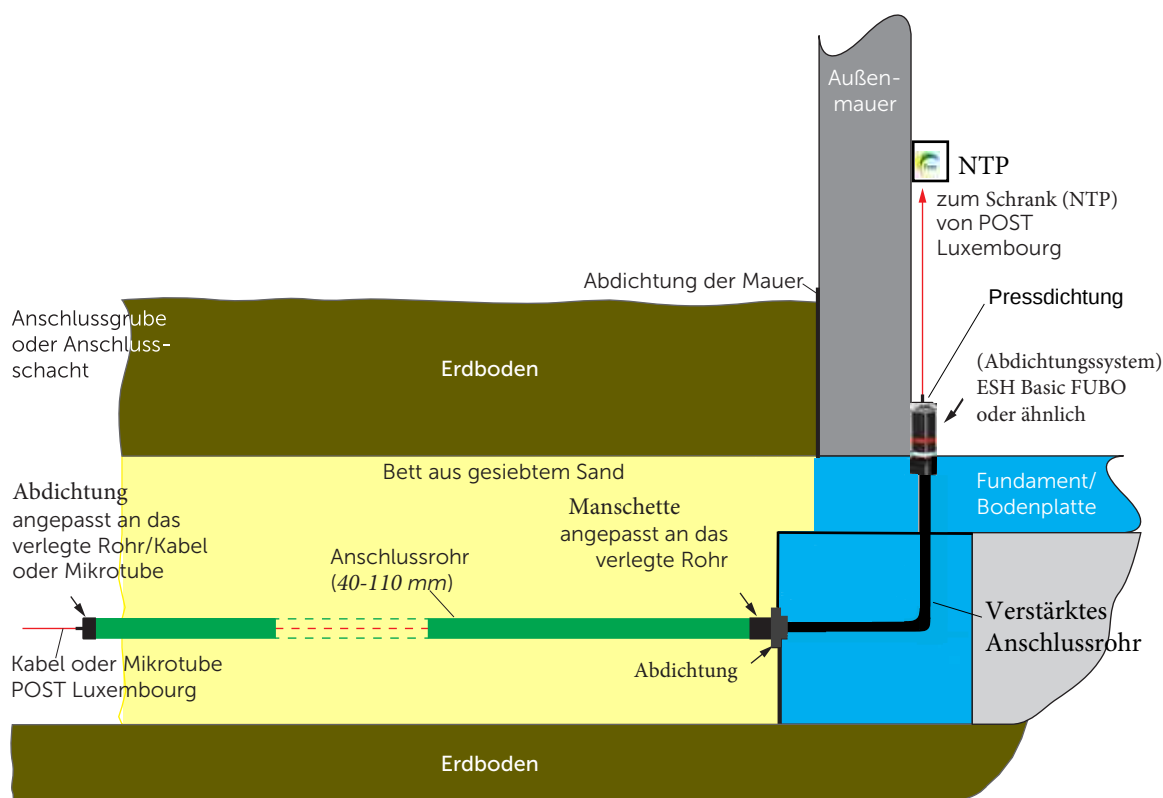
Abb. 6 Einführung der Kabel/Microtube ins Gebäude durch die Bodenplatte
