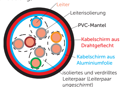
Abbildung 28 Netzkabel Kat.5e SF/UTP 4x2 (Paare nicht geschirmt) für die Horizontalverkabelung
