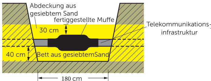
Abb. 8 Fertiggestellte Muffe in der Anschlussgrube mit Schutz des Kabels und der Muffe mit einer Abdeckung aus gesiebttem Sand
