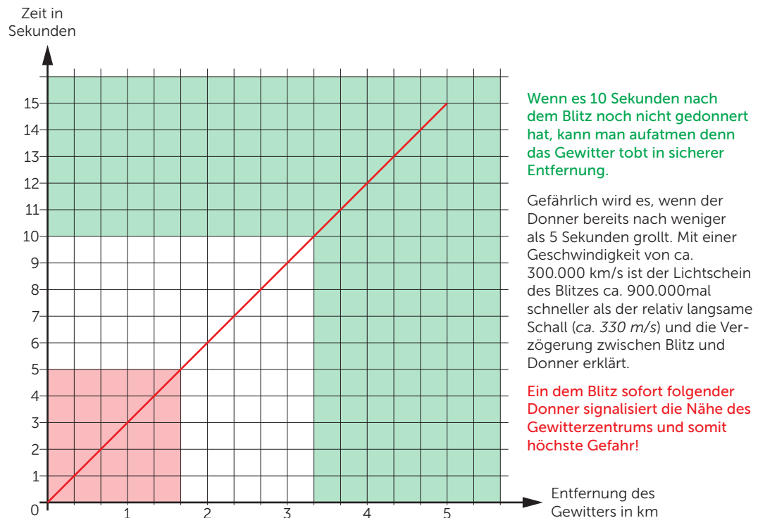
Abbildung 14 Grafik über die Berechnung der Entfernung eines Gewitters anhand des Zeitintervalls zwischen Blitz und Donner
