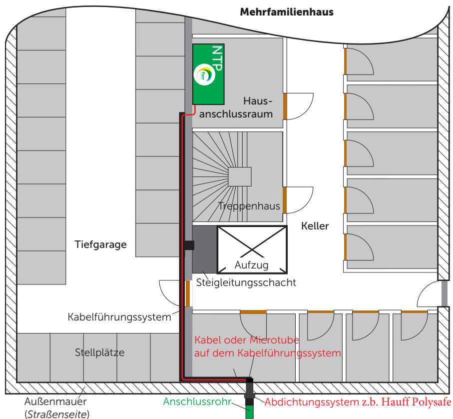
Abb. 2 Hausanschlussraum ohne direkten Kontakt zum Anschlussrohr
