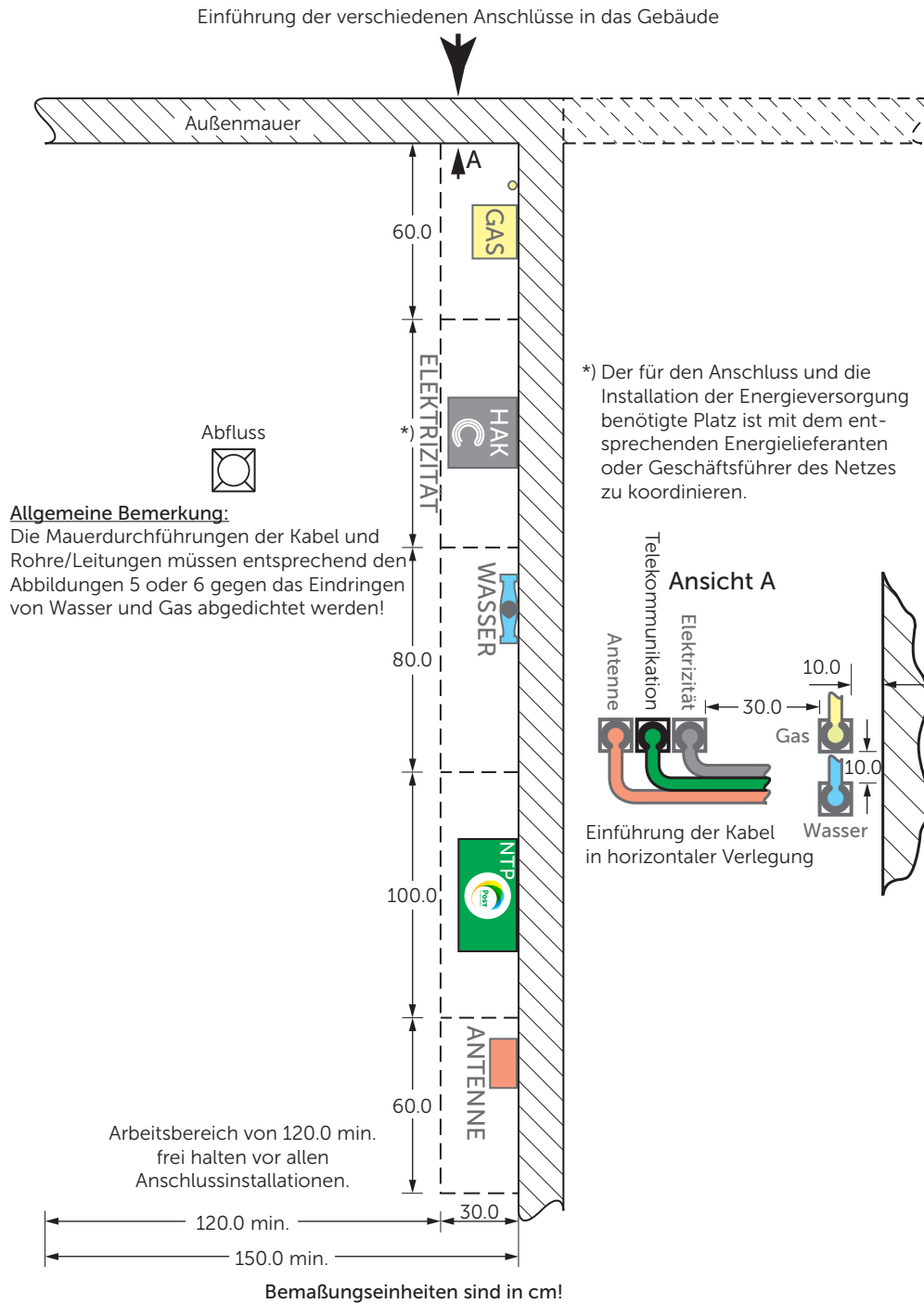
Abb. 12 Anschlussstyp für ein Mehrfamilienhaus bis 3 Wohneinheiten – Beispiel einer Ausführung Hausanschlussraum Benutzung 1 Seite – Außenmauer auf der Strassenseite
