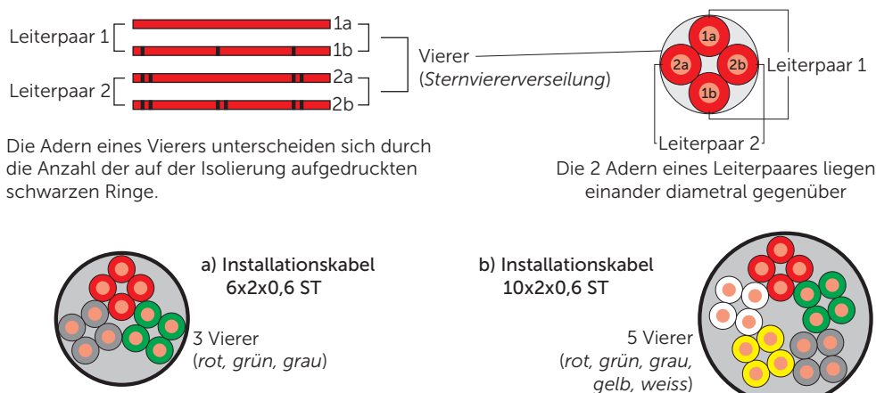
Abb. 31 Installationskabel Kat.3 mit 6 und 10 Leiterpaaren und Kennzeichnung der Leiter im Vierer (Sternviererverseilung)
