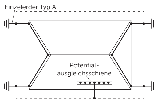
Abb. 16 Erdungsanlage Typ A, Einzelerder
