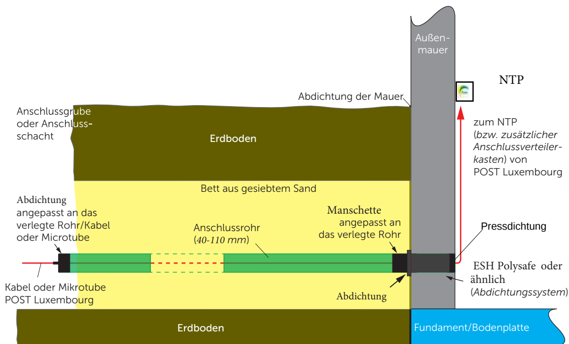
Abb. 5 Einführung der Kabel/Microtube ins Gebäude durch die Außenmauer
