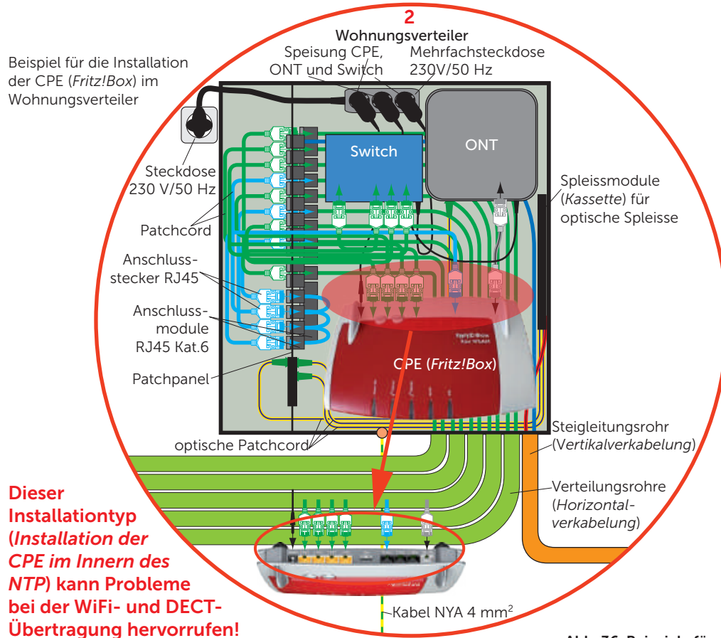
Abb. 36 Beispiele für den Anschluss und die Installation des NTP
