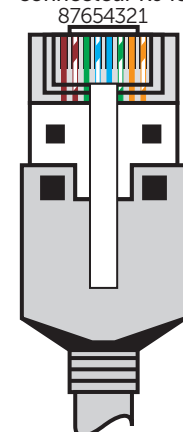
Abb. 30 Stecker und Anschlussmodul RJ45
