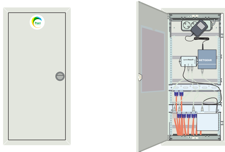
Abb. 25 In die Mauer eingelassener Wohnungsverteiler ( links: geschlossen; rechts: geöffnet )
