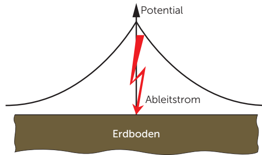
Abbildung 15 Potentialverteilung (Potentialtrichter) bei der punktförmigen Einleitung eines Stromes in das Erdreich
