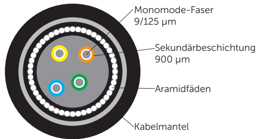
Abb. 26 Glasfaserkabel (4 Fasern) für die Vertikalverkabelung
