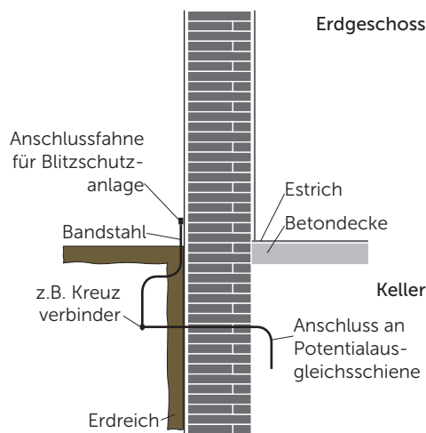
Abb. 18 Erdungsanlage Typ B, Ringerder
