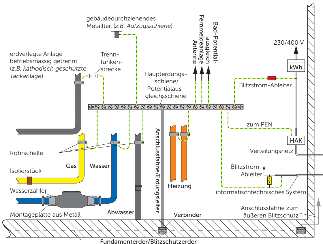
Abbildung 20 Prinzip des Blitzschutz-Potentialausgleiches bestehend aus Blitzschutz- und Schutzpotentialausgleich
